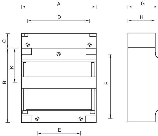
Verdeler VKS21S, incl. buisvoerstuk
